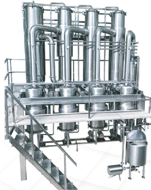
Evaporatör (Vakum) / Evaporator (Vacuum) Вакуумный испаритель / جهاز التكتيف
