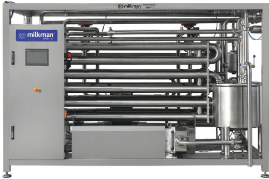
Tubular Pastörizatör / Tubular Pasteurizer Трубчатый пастеризатор / البسترة الأنبوبية
