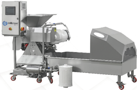
Mozerella Ünitesi / Mozzarella Unit
