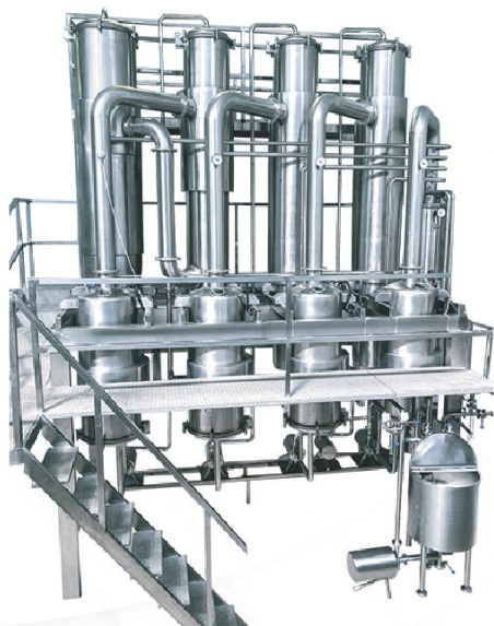
Evaporatör (Vakum) / Evaporator (Vacuum) Вакуумный испаритель / جهاز التكثيف
